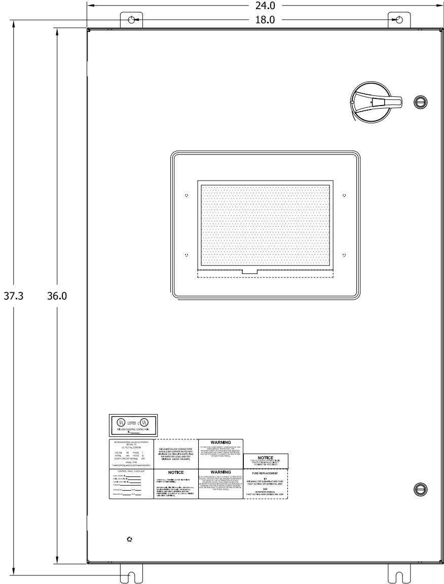
TYPE 4 ENCLOSURE CARBON STEEL, PAINTED BLUE 36"(H) X 24" (W) X 10" (D)
